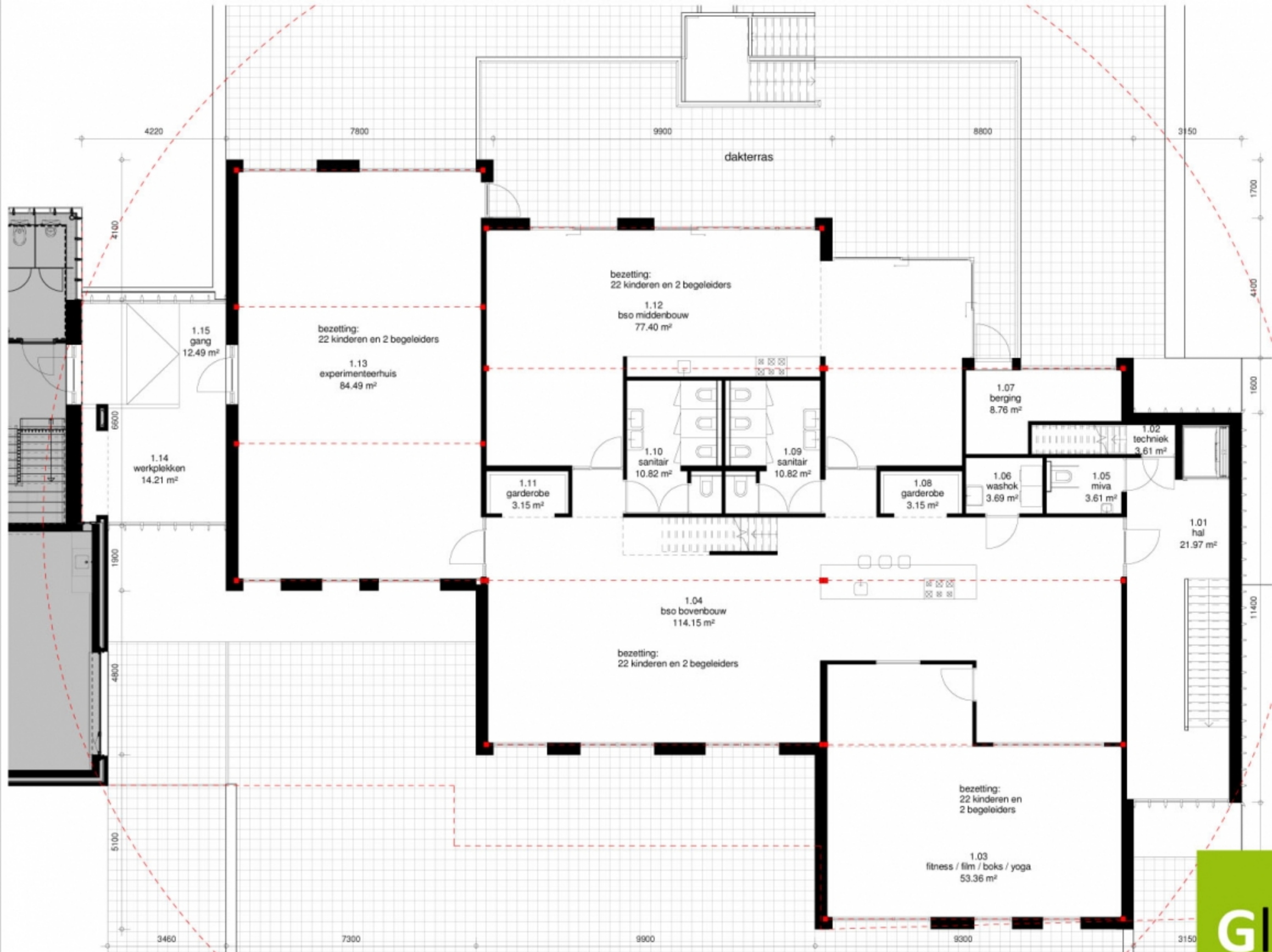
verdieping 1:100
